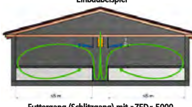
Futtergang (Schlitzgang) mit »ZED« 5000
