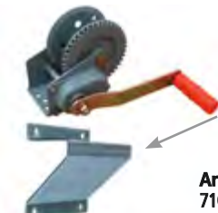
Auslöse-Seilwinde, für Dosierbehälter 500 kg Zugkraft selbsthemmend mit Wandhalterung
